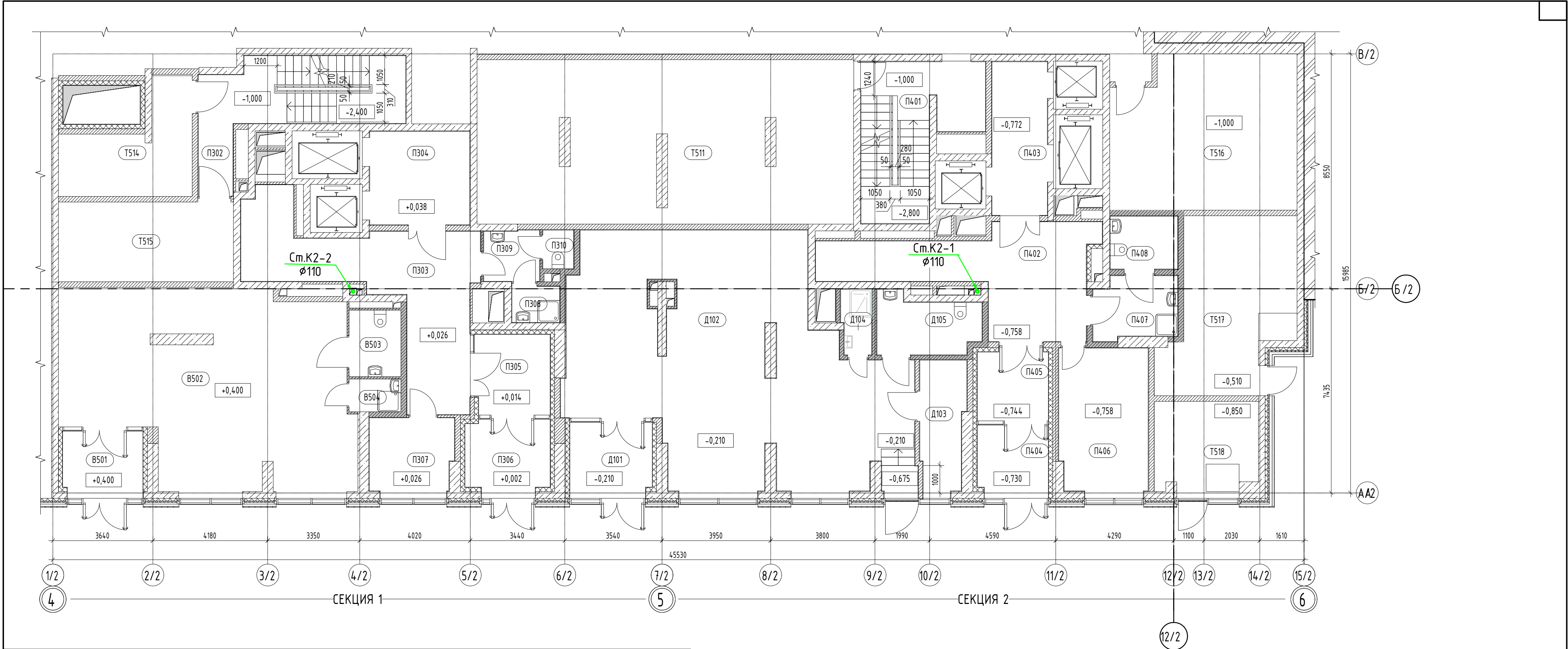
Экспликация помещений 1 этажа
