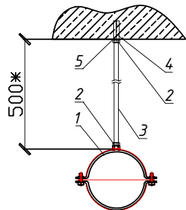
Подвес чугунных труб СМЛ ф100
