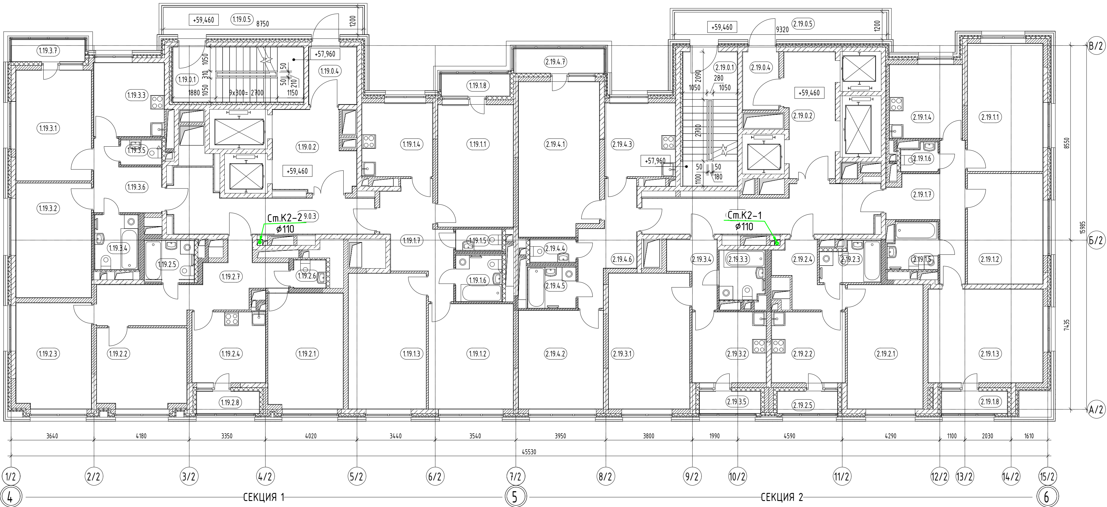
Экспликация помещений 19 этажа
