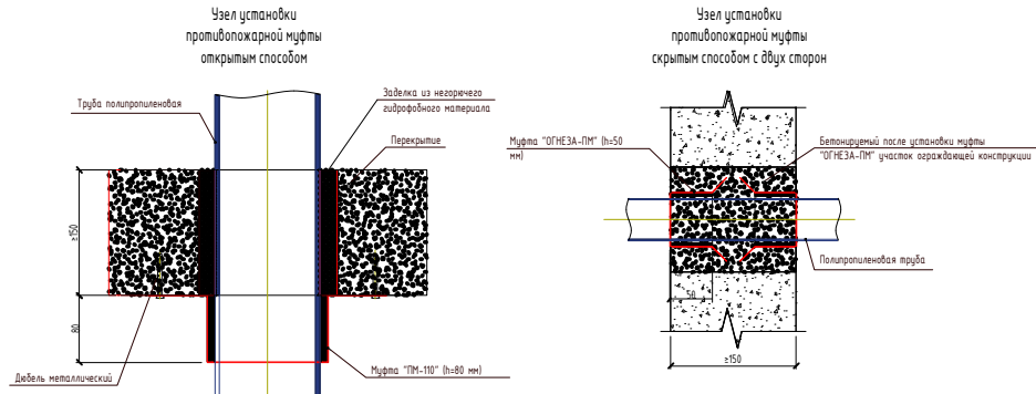
Крепление канализационной трубы Ø110 к стене
