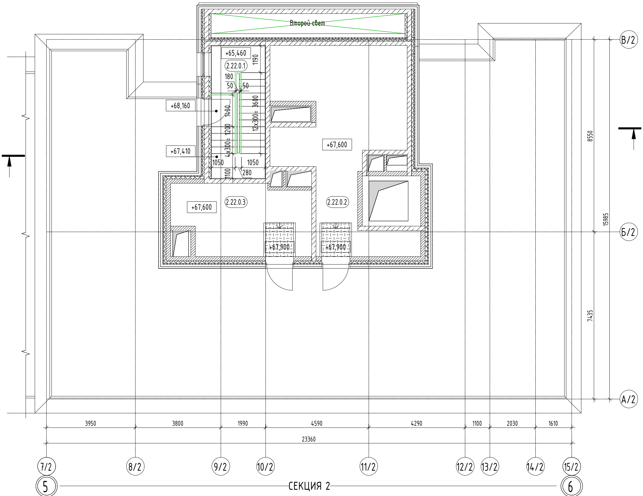
Маркировочный план на отм. +67,600
