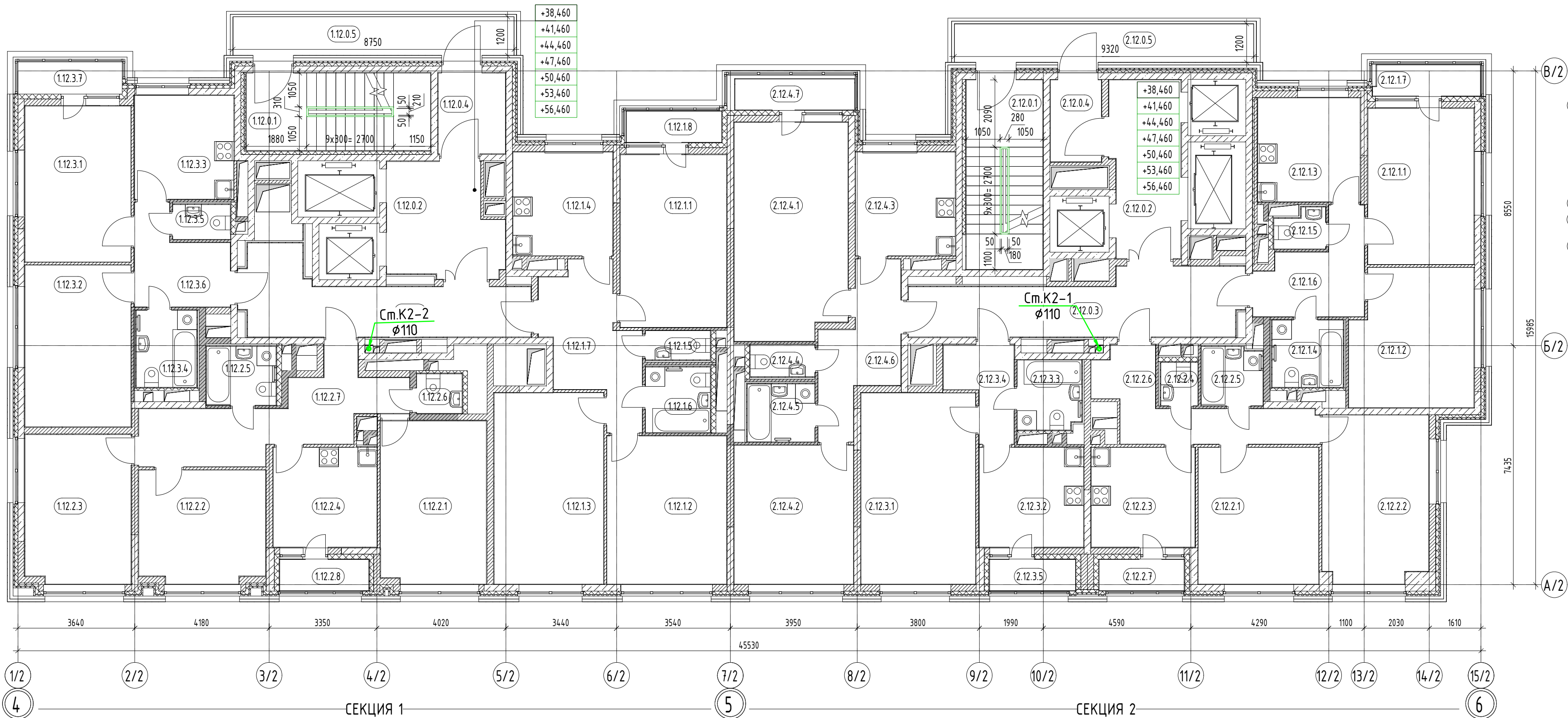
Экспликация помещений 12-18 этажей
