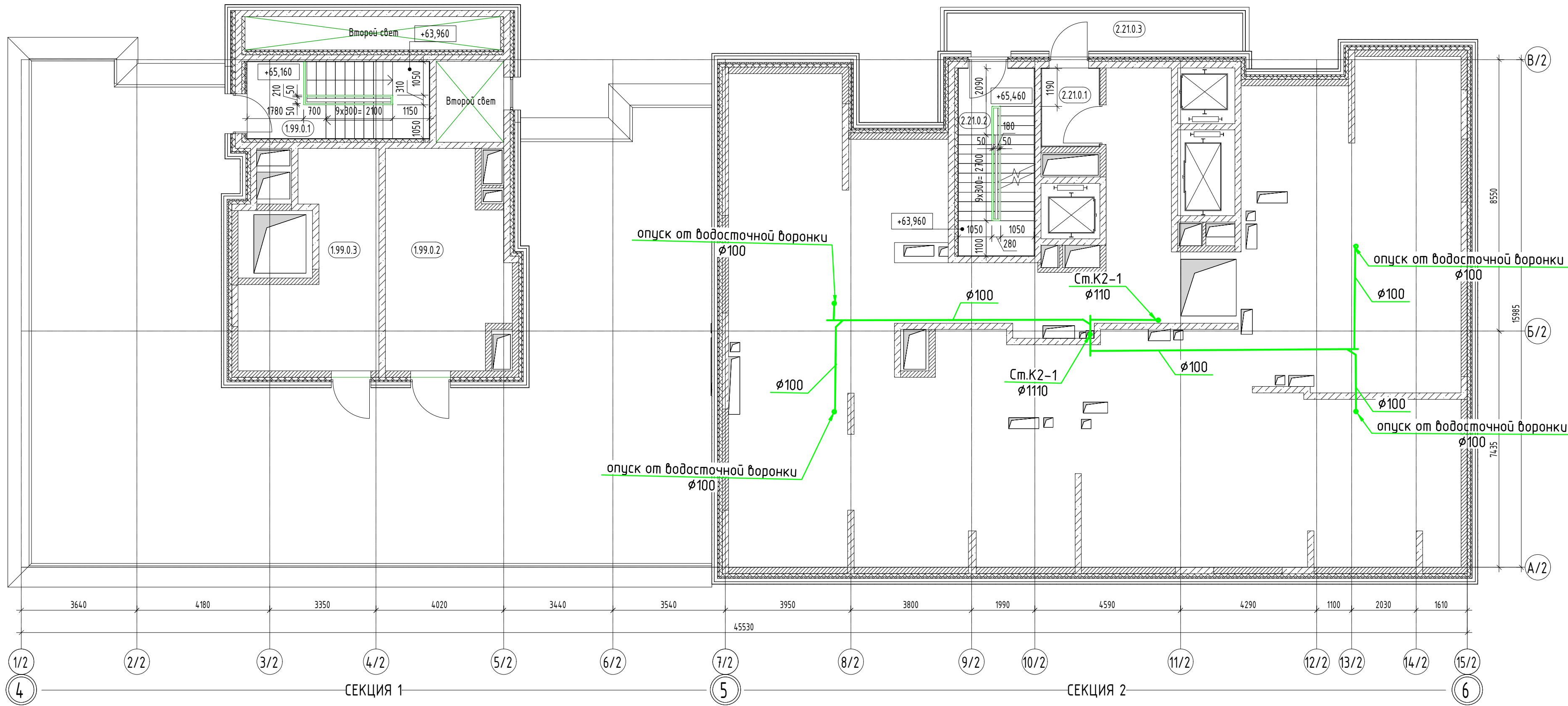
Маркировочный план на отм. +64,580; +65,460
