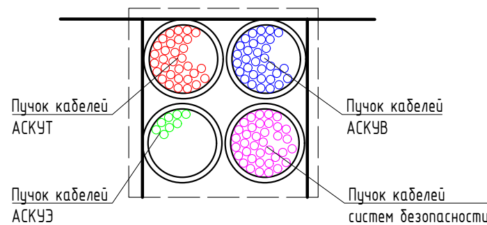
Типовой эскиз заполнения стояка СС
