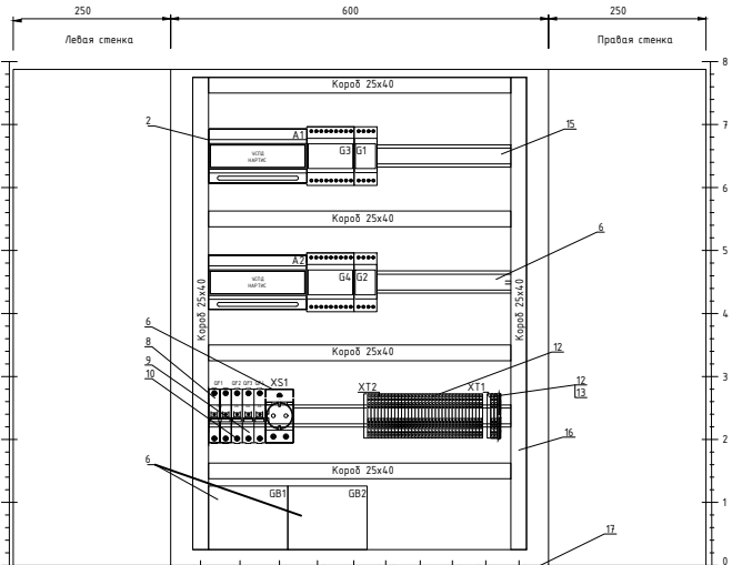
Вид на внутренние плоскости (развернуто)
