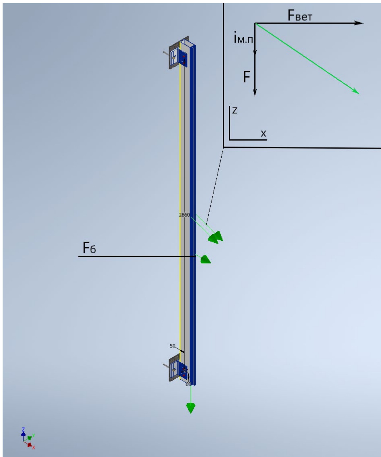
Рисунок 2.6. Схема действующих нагрузок. Общий вид.
