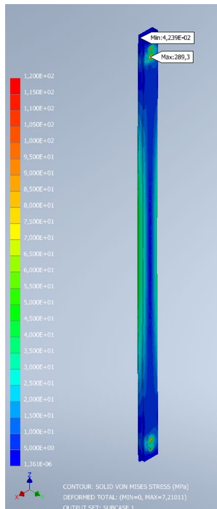
Рисунок 3.2. Изополя максимальных эквивалентных напряжений вертикального профиля.
