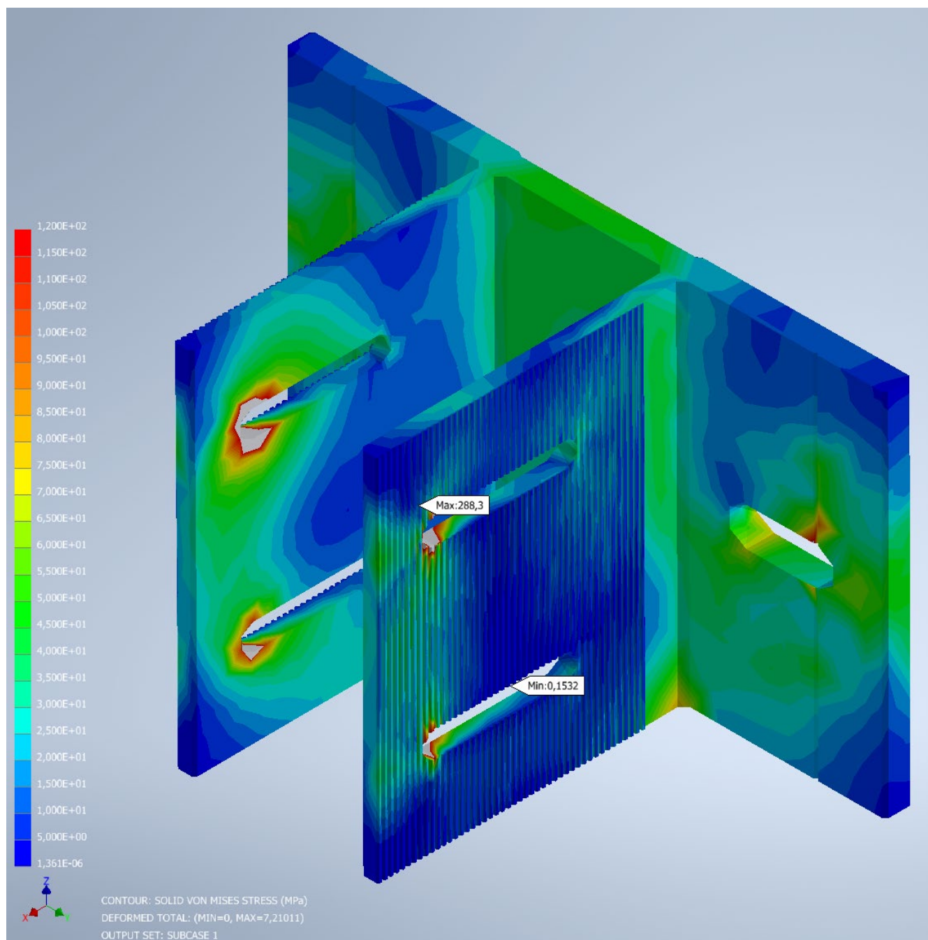
Рисунок 3.4. Изополя максимальных эквивалентных напряжений опорного кронштейна.
