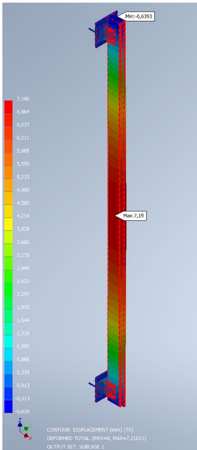
Рисунок 3.6. Участок подсистемы. Перемещения вдоль оси X.
