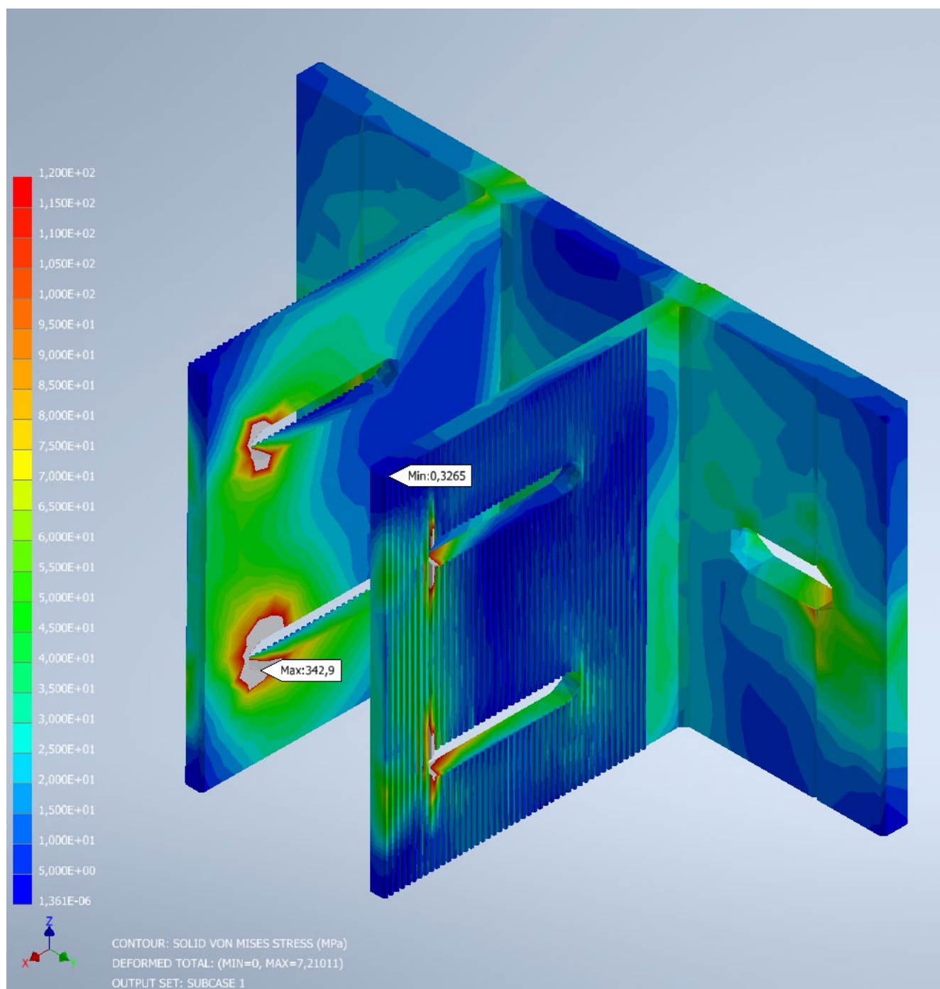
Рисунок 3.1. Изополю максимальных эквивалентных напряжений несущего кронштейна.
