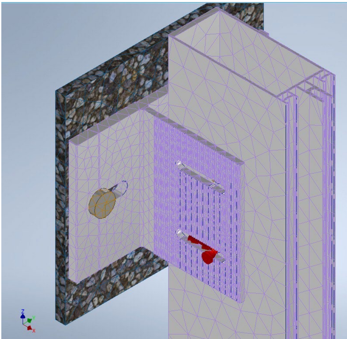
Рисунок 2.5. Сетка конечных элементов. Вид на несущий кронштейн.
