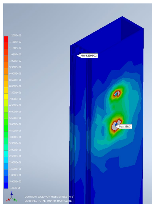
Рисунок 3.3. Изополя максимальных эквивалентных напряжений вертикального профиля. Вид на зону смятия.
