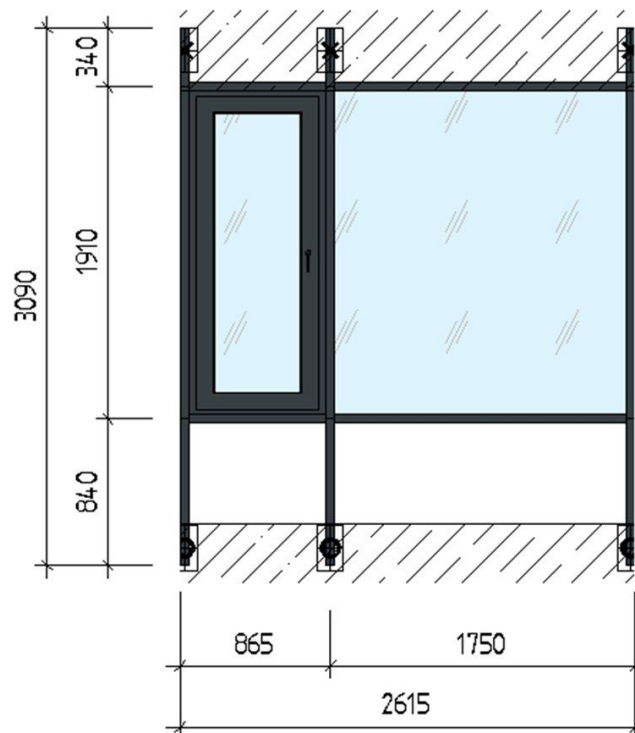
Рисунок 2.1. Конструкция витражного блока. Вид спереди.
