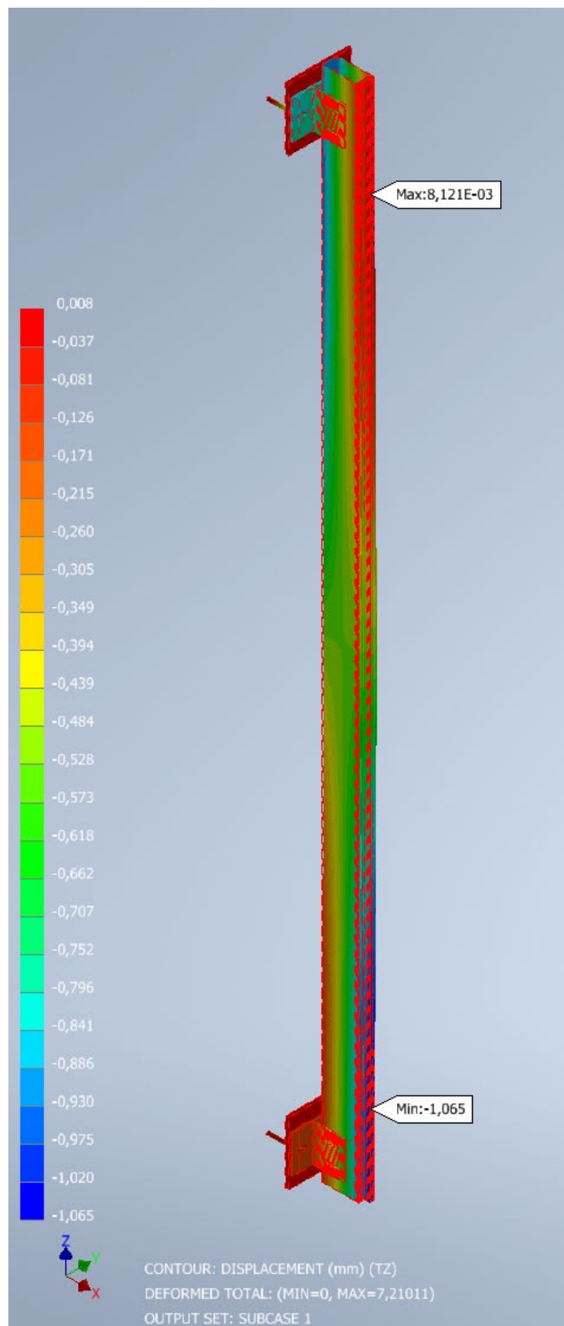
Рисунок 3.8. Участок подсистемы. Перемещения вдоль оси Z.
