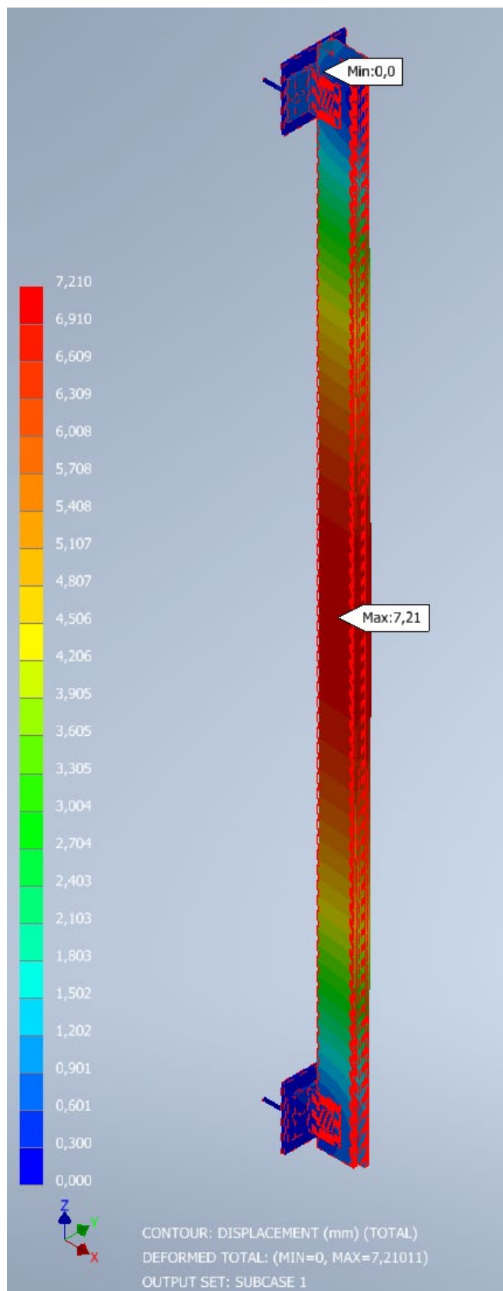
Рисунок 3.5. Участок подсистемы. Общие перемещения.
