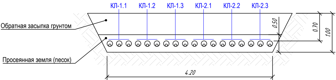
Схема укладки кабелей
