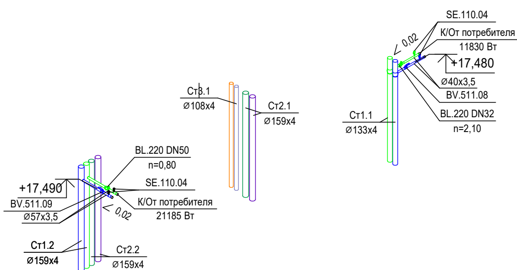
Схема системы холодоснабжения 5 этажа (14,700)
