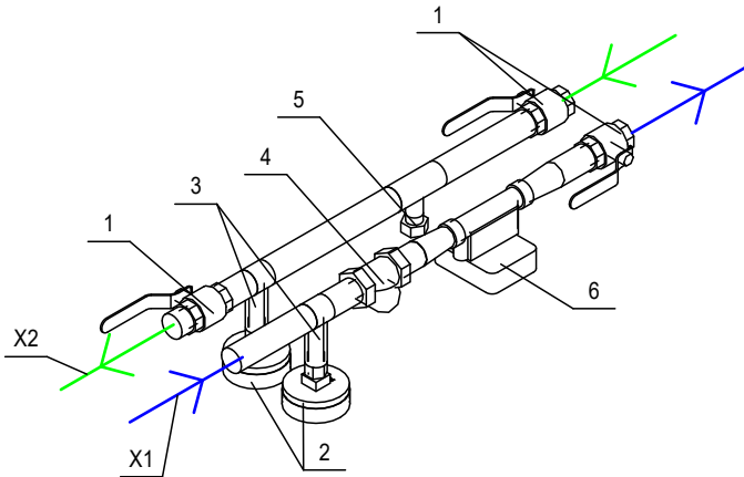
Узел учета тепловой энергии D20-D40
