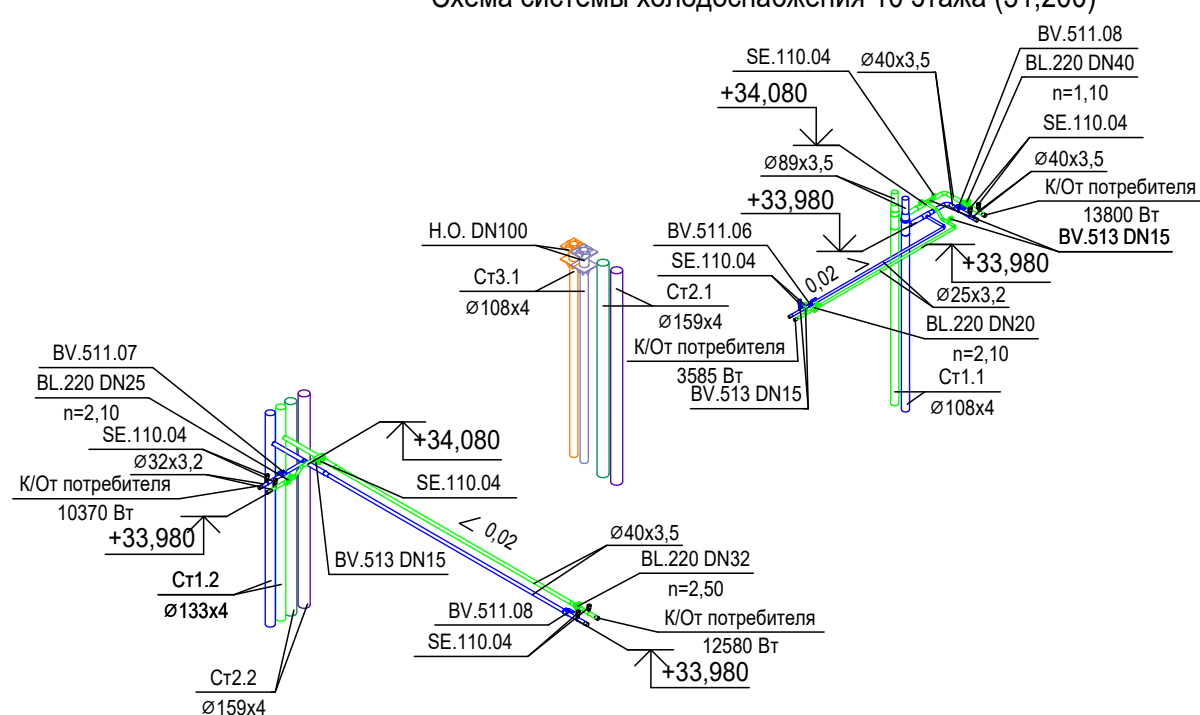
Схема системы холодоснабжения 10 этажа (31,200)
