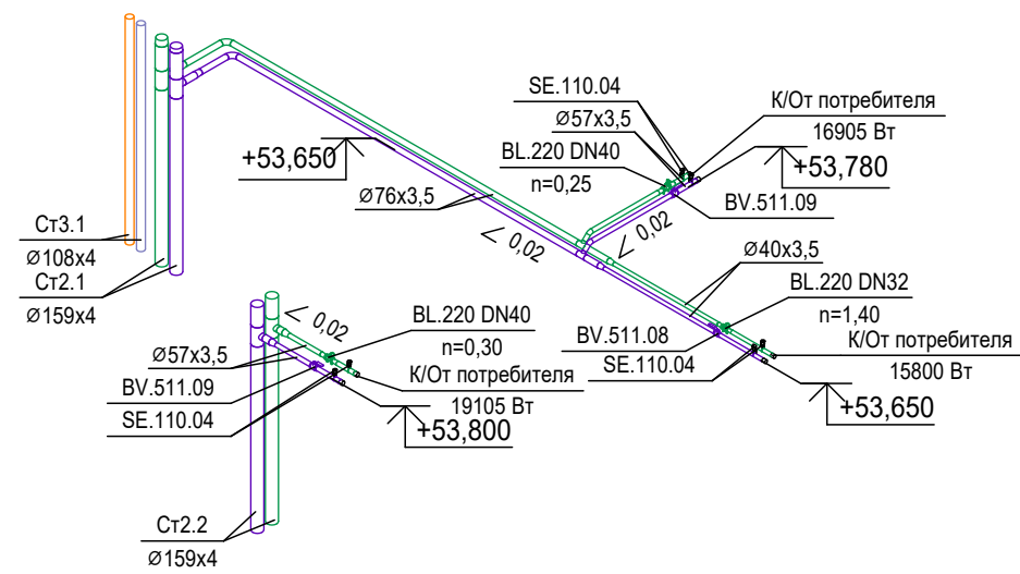
Схема системы холодоснабжения 16 этажа (51,000)
