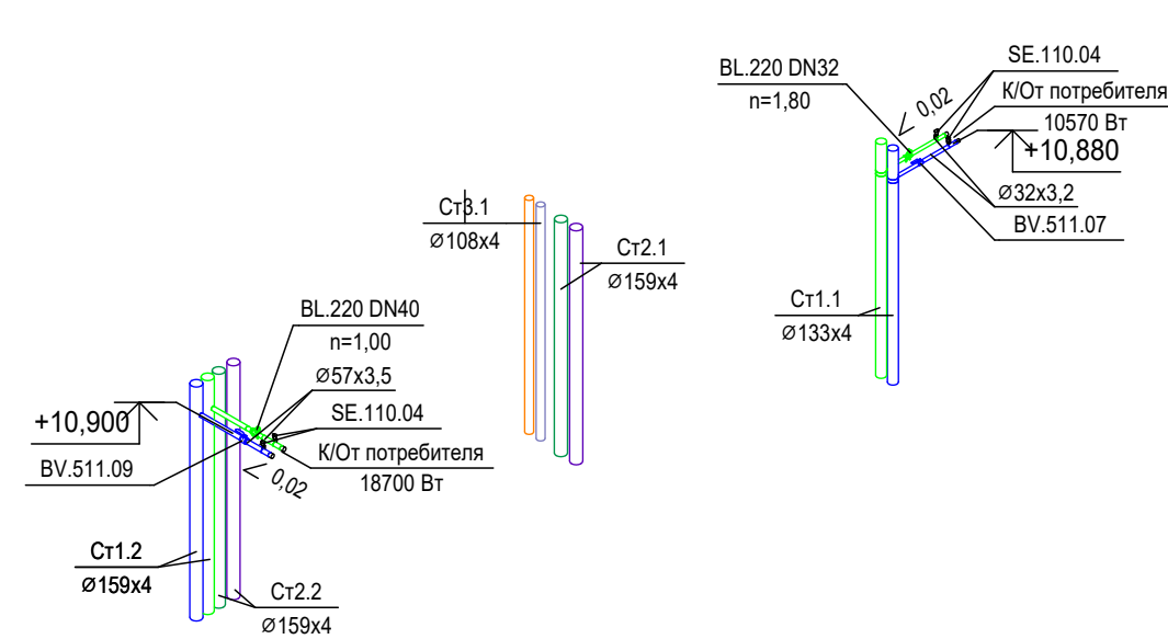
Схема системы холодоснабжения 3 этажа (8,100)
