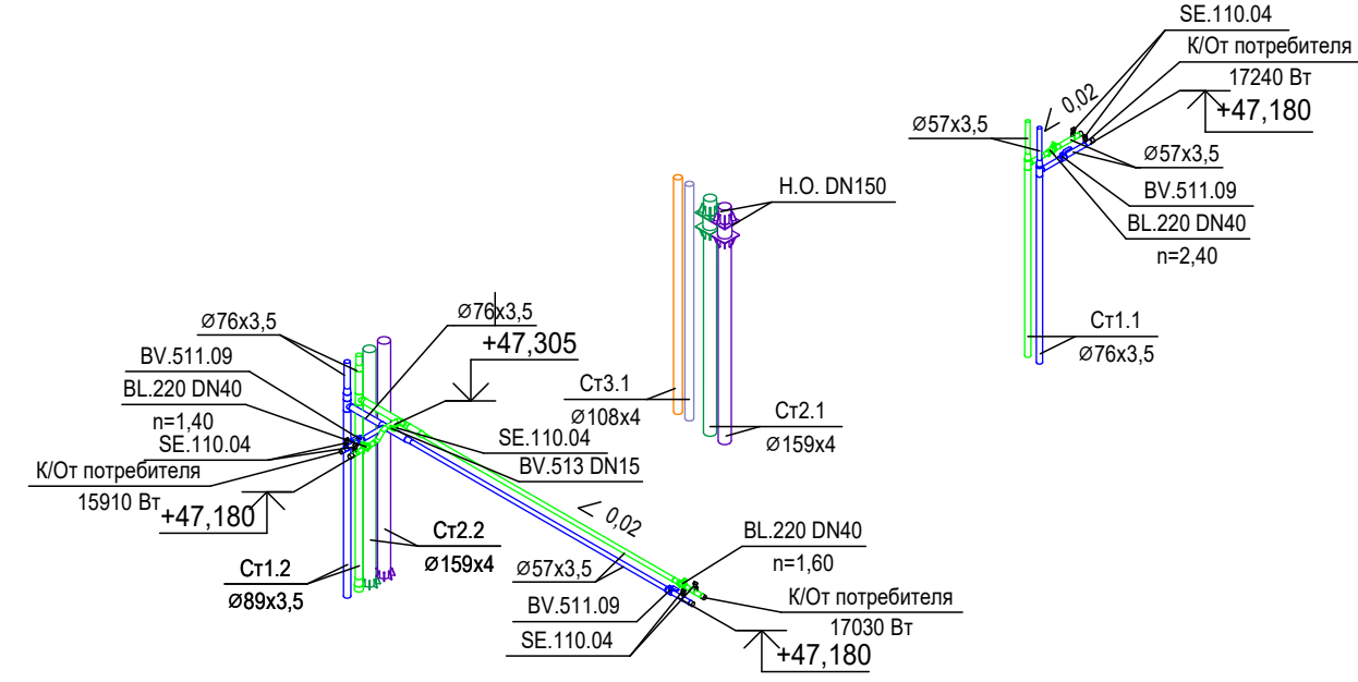
Схема системы холодоснабжения 14 этажа (44,400)
