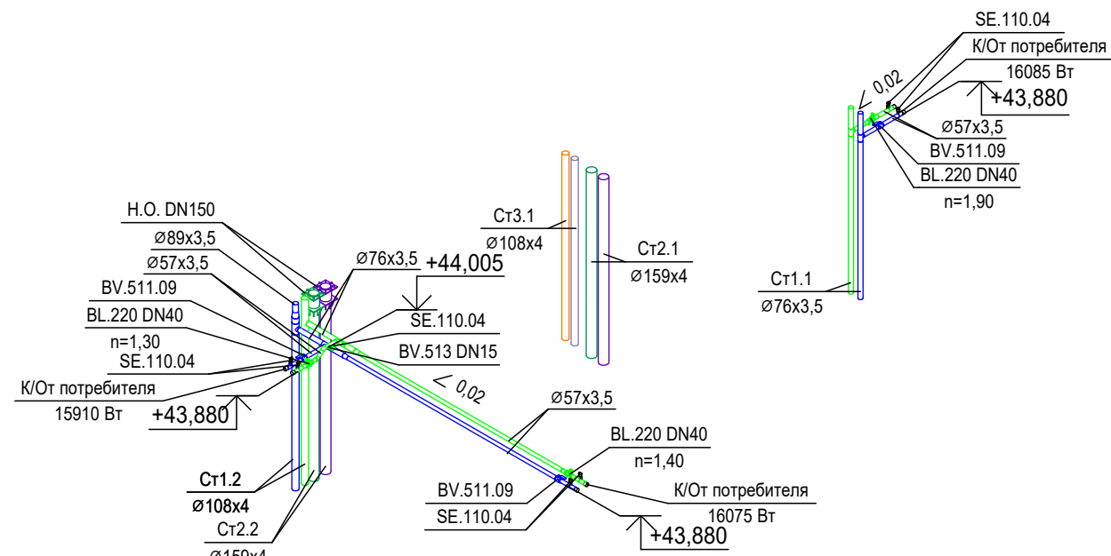
Схема системы холодоснабжения 13 этажа (41,100)
