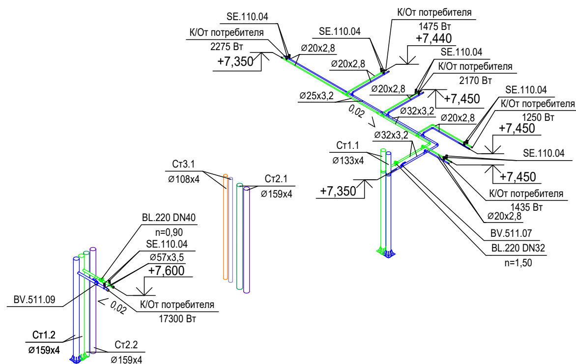
Схема системы холодоснабжения 2 этажа (4,800)
