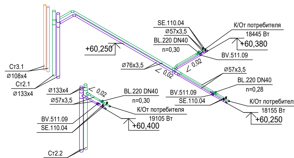
Схема системы холодоснабжения 18 этажа (57,600)
