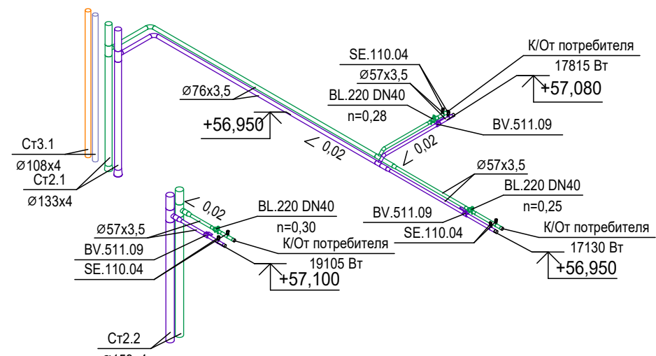
Схема системы холодоснабжения 17 этажа (54,300)
