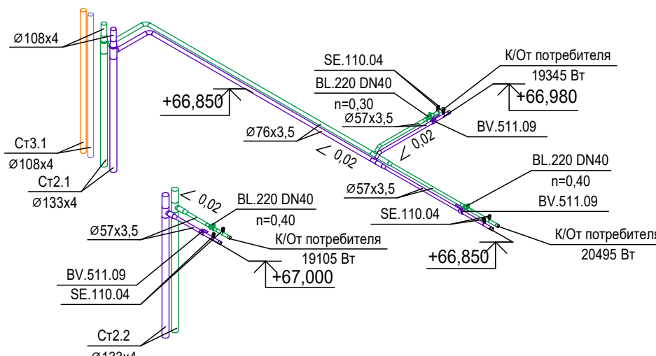
Схема системы холодоснабжения 20 этажа (64,200)
