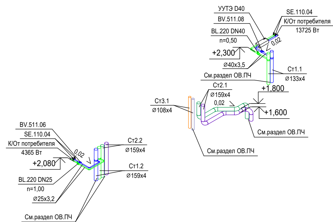
Схема системы холодоснабжения 1 этажа (-2,700)
