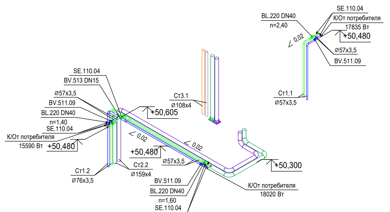
Схема системы холодоснабжения 15 этажа (47,700)
