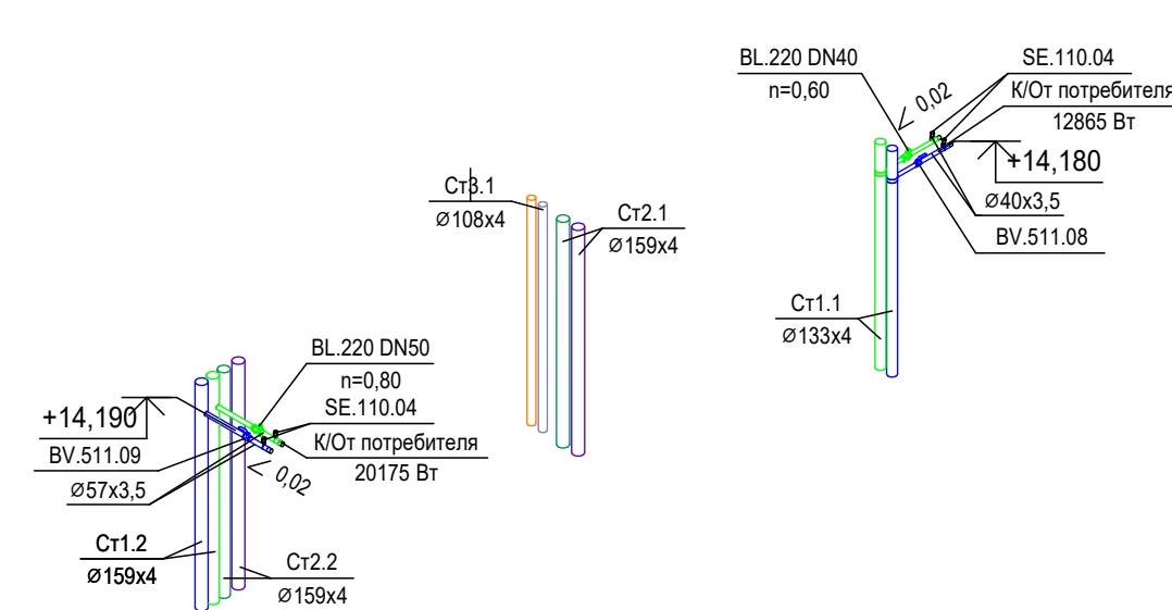
Схема системы холодоснабжения 4 этажа (11,400)
