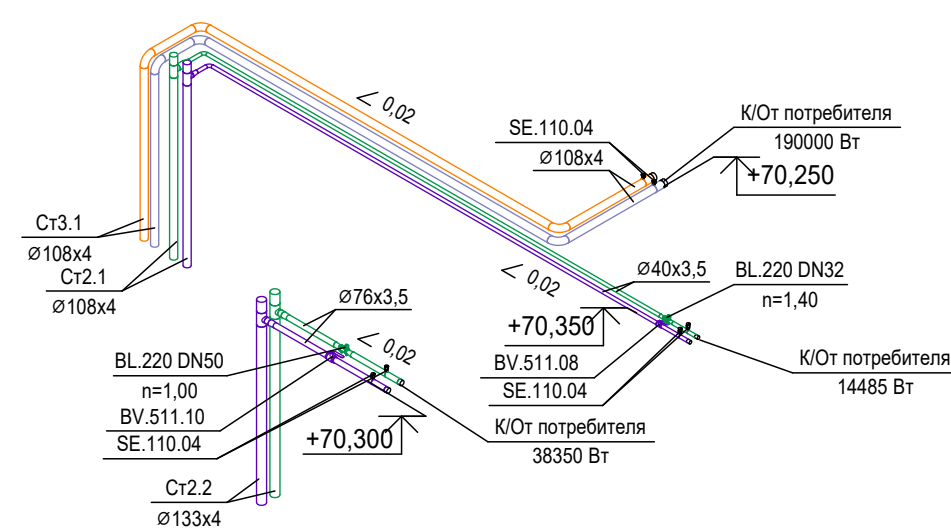
Схема системы холодоснабжения 21 этажа (67,500)
