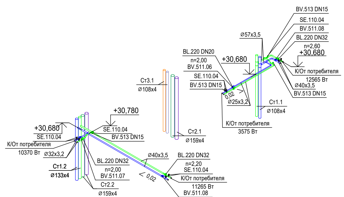
Схема системы холодоснабжения 9 этажа (27,900)
