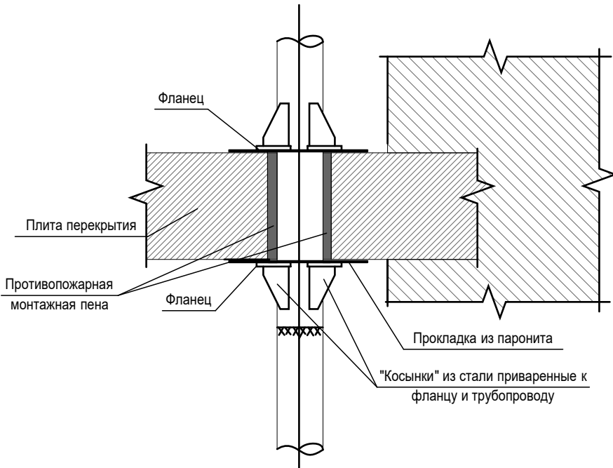
Узел неподвижной опоры
