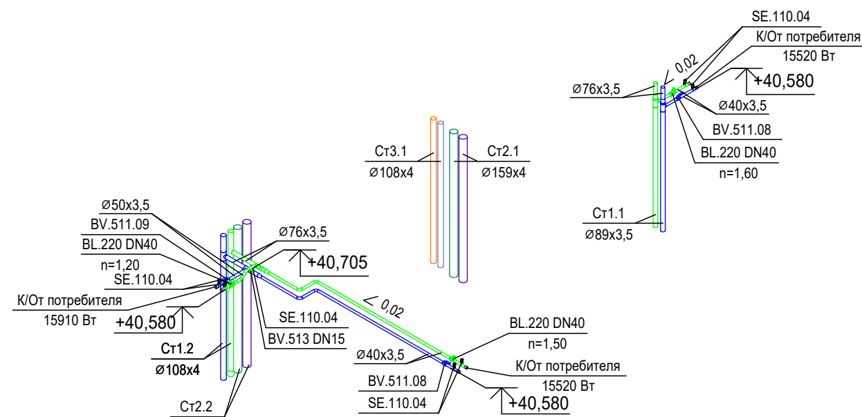
Схема системы холодоснабжения 12 этажа (37,800)
