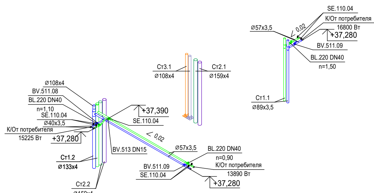
Схема системы холодоснабжения 11 этажа (34,500)
