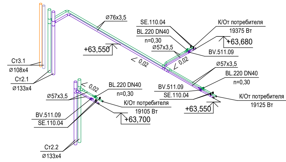
Схема системы холодоснабжения 19 этажа (60,900)
