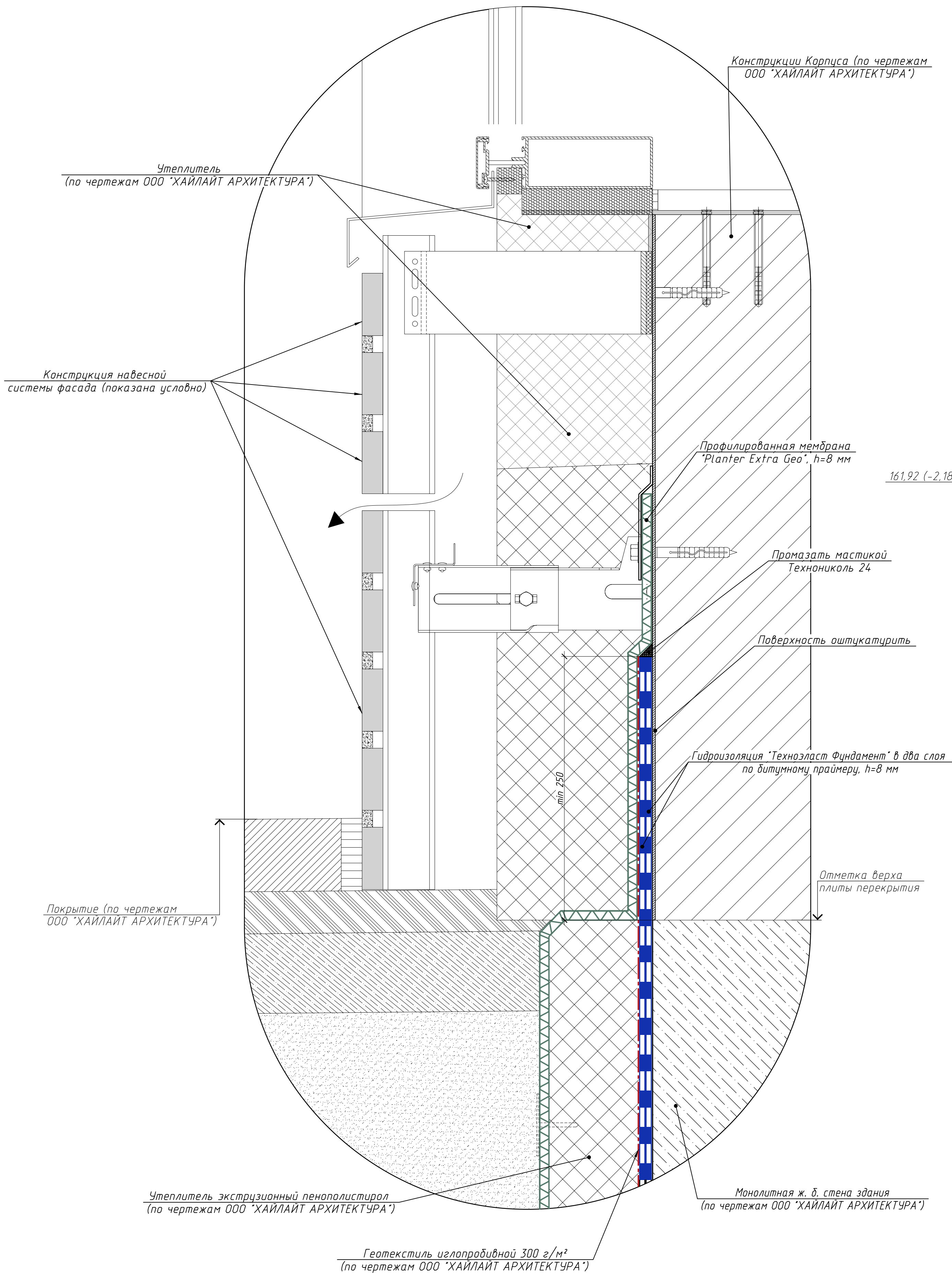
Узел устройства завершающего ряда гидроизоляции (1:2,5)
