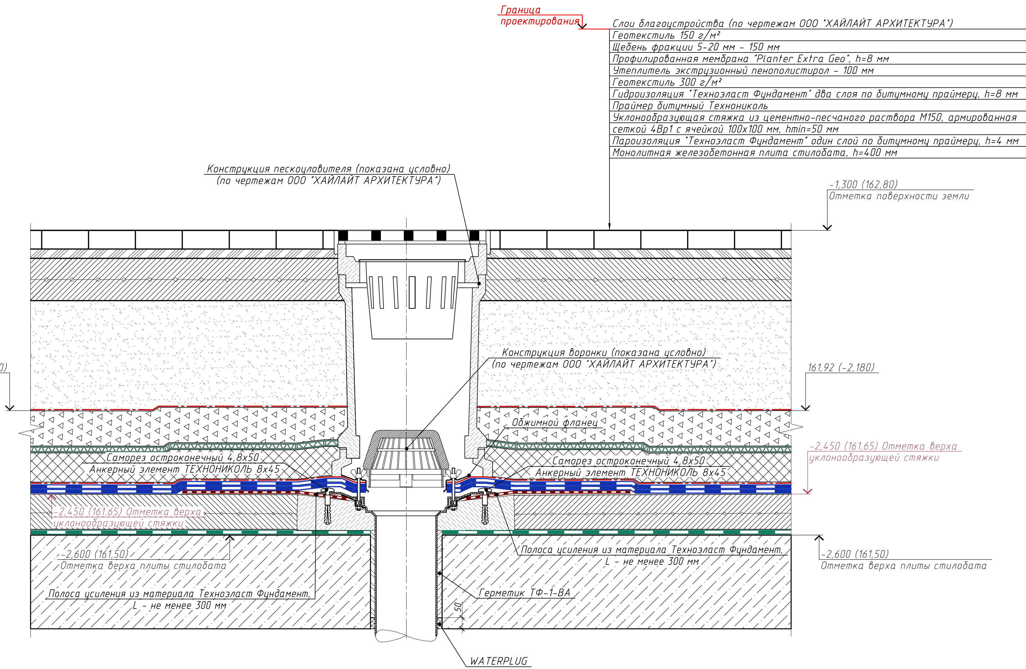
Разрез 11 - 11. Принципиальный узел гидроизоляции кровельной воронки
