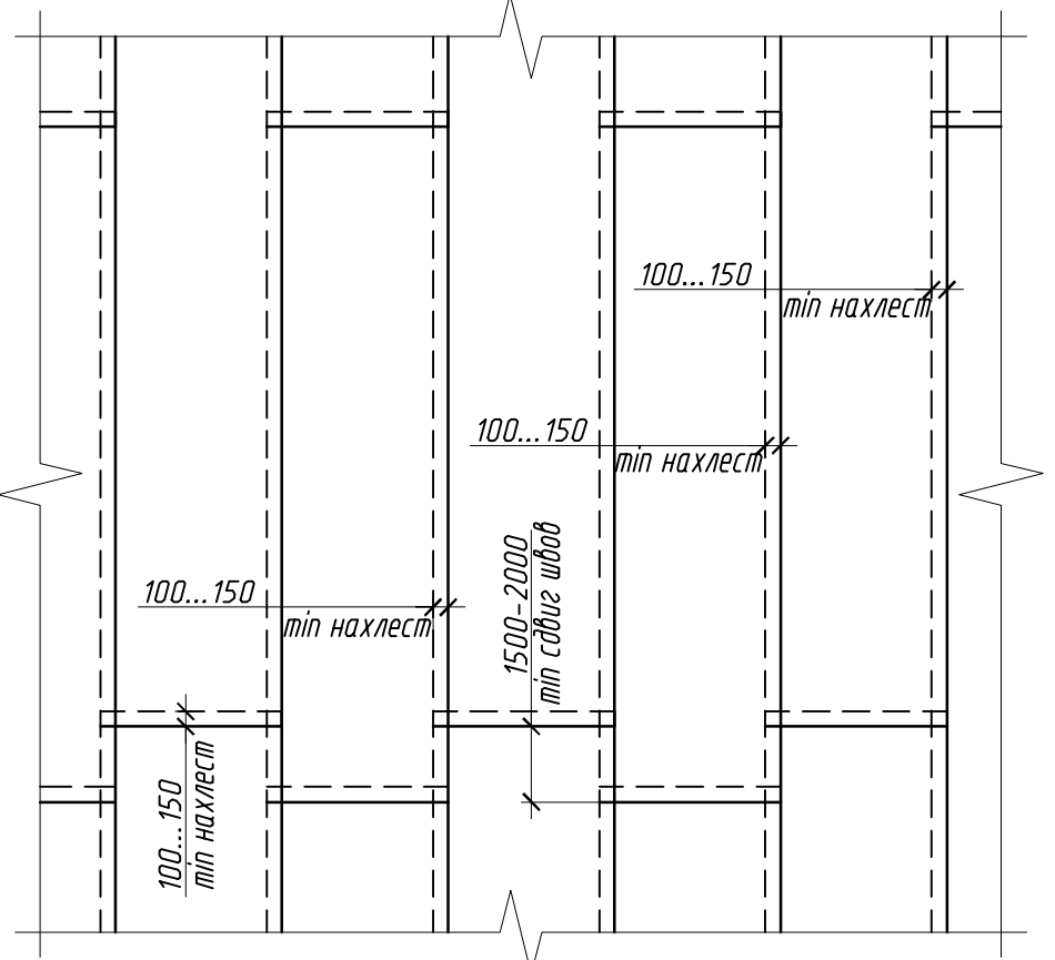
Фрагмент раскладки материала "Planter Extra Geo"
