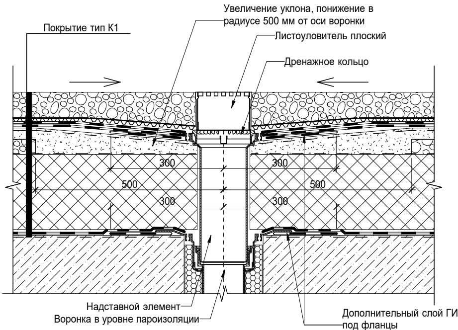
Кровля. Водосточная воронка
