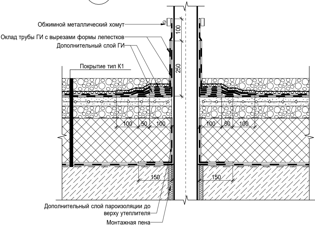
Кровля. Фановый стояк ВК
